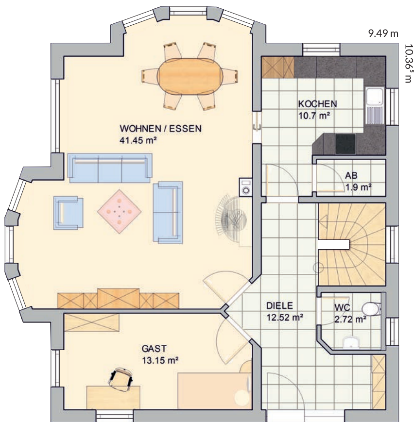
Erdgeschoss
